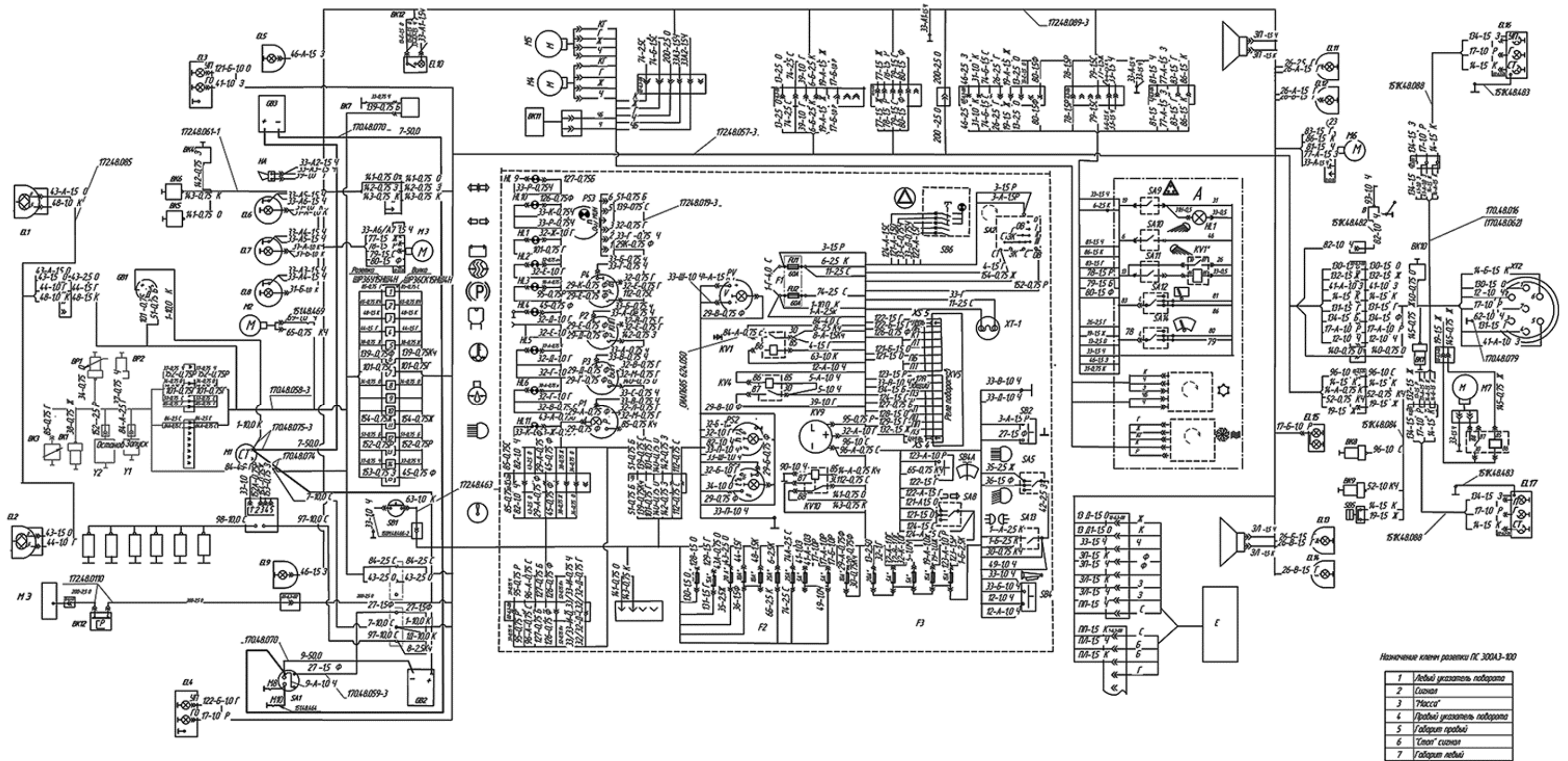
Рисунок 61 – Схема электрическая соединений электрооборудования трактора ХТЗ – 17021
